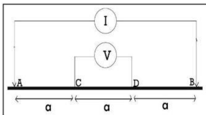
Gambar 2. Skema survei geolistrik dengan metode Schlumberger
