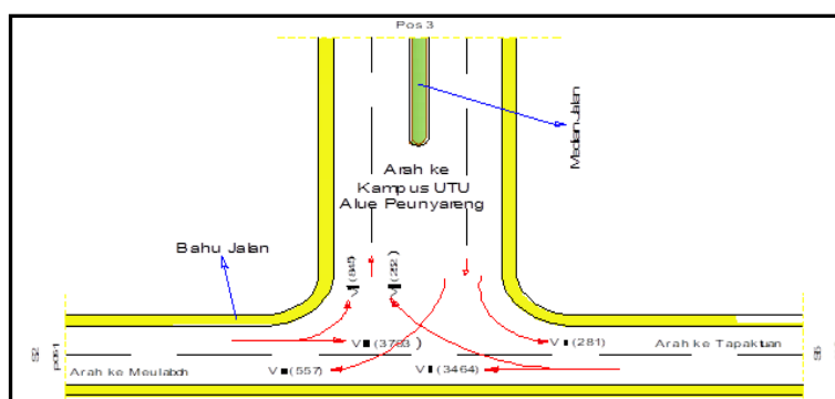
Gambar 2. Sketsa Pergerakan Simpang Tiga Gunong Kleng
